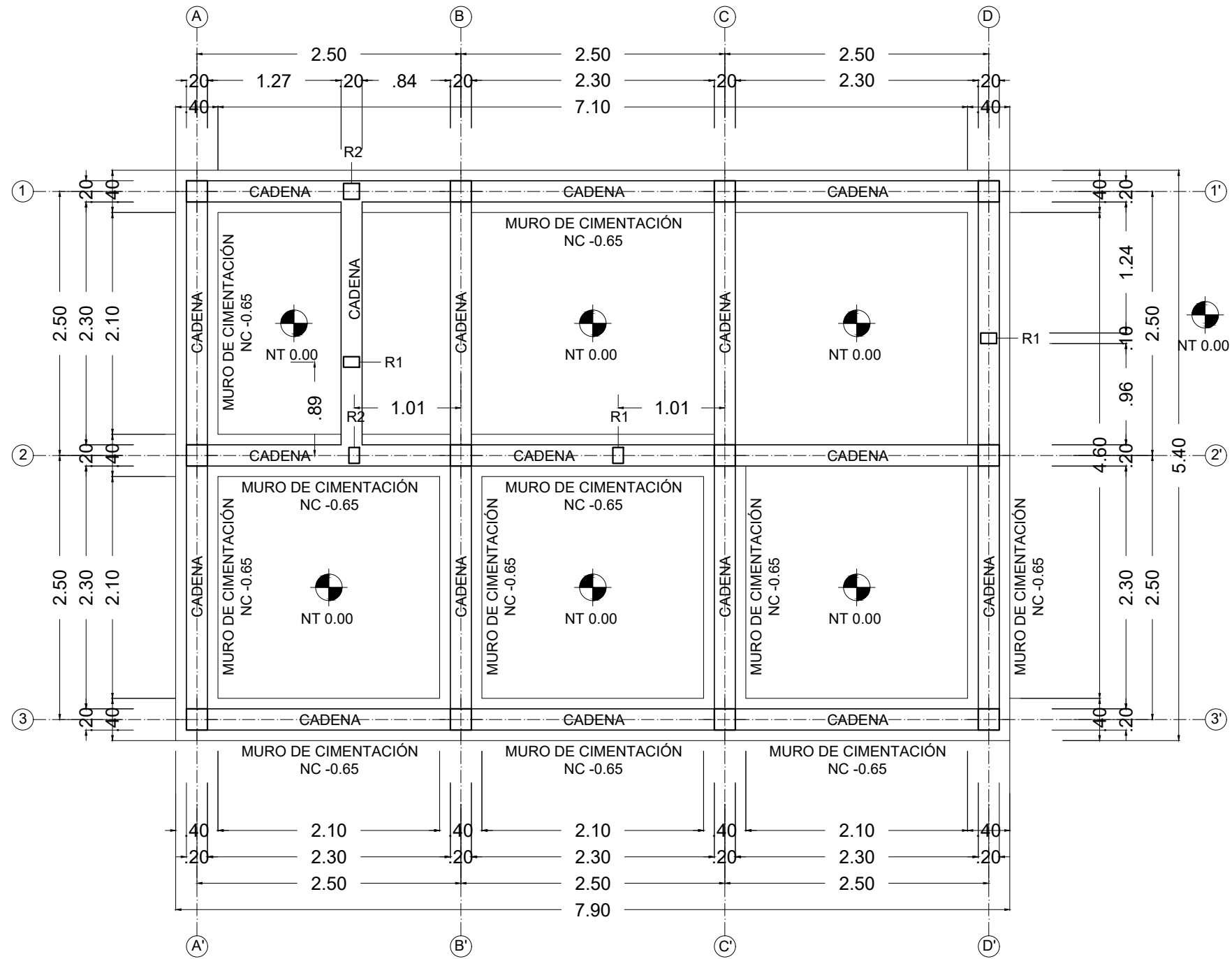
PLANTA DE CIMENTACIÓN
